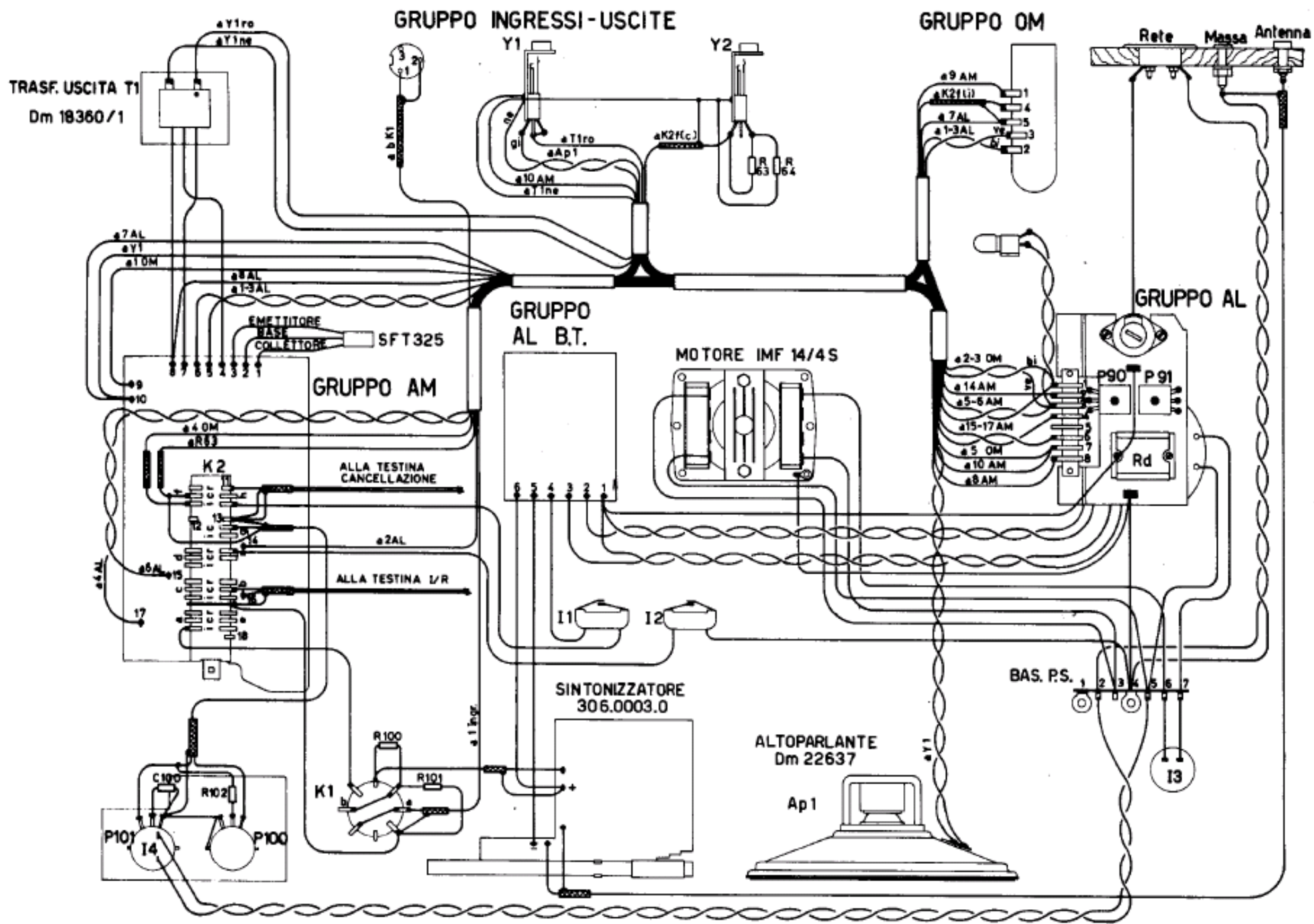
- Cablaggio Radiorenas PR 2.
